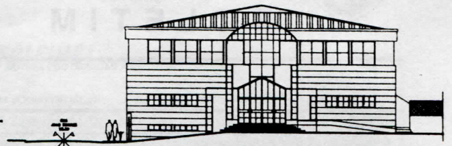
Alçado Sul
