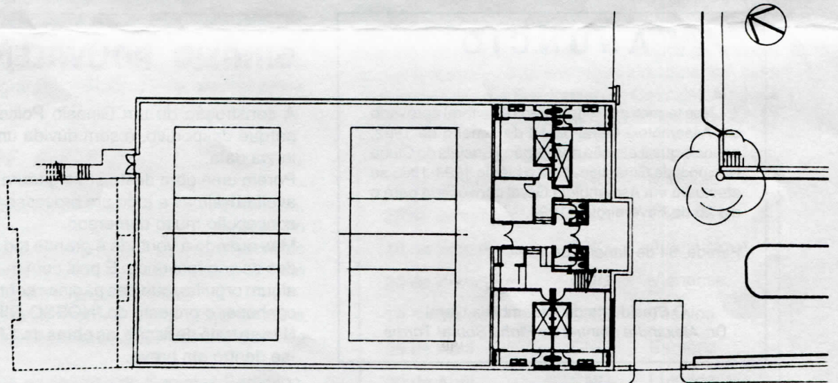
Planta ao Nivel do Campo de Jogos
